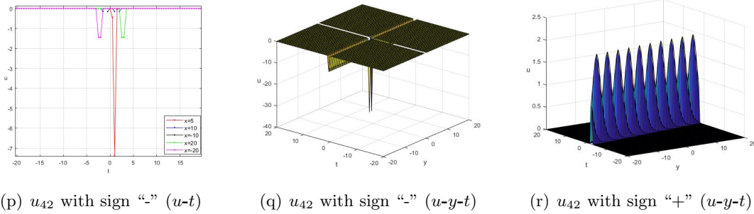
Fig.6 a_4 = k_3 = k_4 = -l_3 = d_3 = d_4 = 1, c_3 = c_4 = -4, a_3 = l_4 = 2, x = z = 0 .
