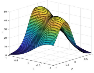
(d) u-z-t with c_3 = -1
