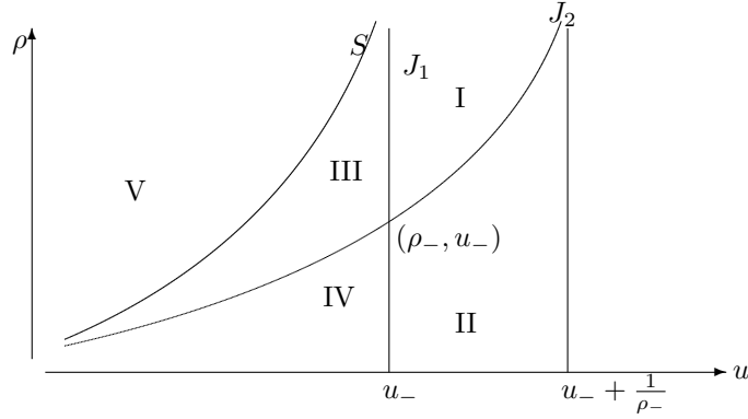
Figure 1. (\rho, u) -plane.
